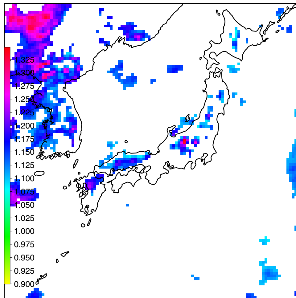
左が50年後の年降水量 / 現在の年降水量，右が100年後の年降水量 / 現在の年降水量 白い部分は「統計的に降水量が増えたり減ったりするとは判断できない」部分
