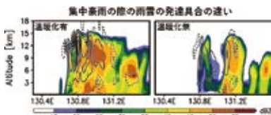
図2 海洋温暖化が集中豪雨に及ぼす影響
