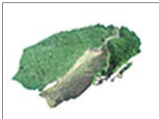
図1 空撮写真から森林の3次元化
