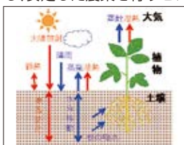
土壌－植物－大気の水・熱循環
