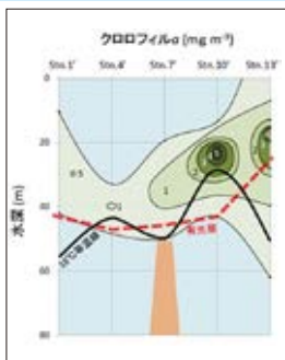
金洲ノ瀬におけるクロロフィルa濃度の断面図
