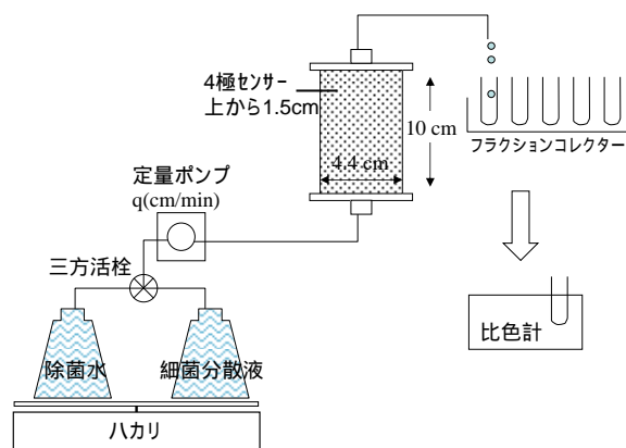
図1 実験装置図
