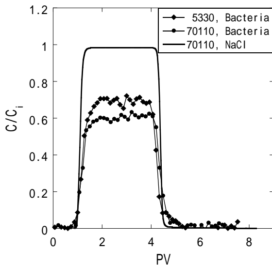
図 2 流出液の PV と相対細菌濃度の関係
