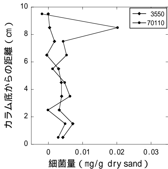
図 3 カラム内に保持された細菌量の垂直分布
