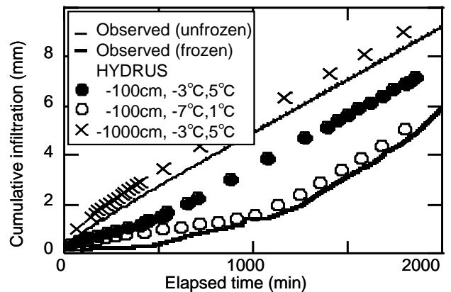
図 3 凍土への浸潤量
