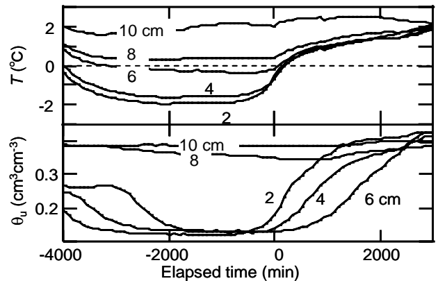
図 1 凍結・浸潤(融解)過程にある土の温度と水分量変化。
