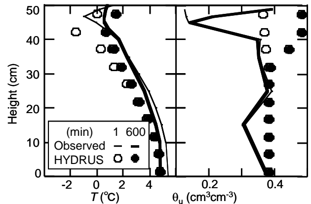
図 2 浸潤(融解)過程にある土の地温分布と液状水量分布
